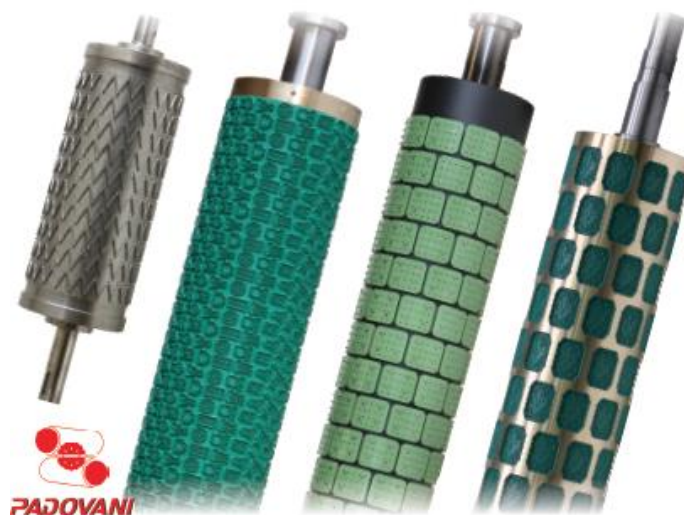
Роторы для сахарного, затяжного печенья и крекера
